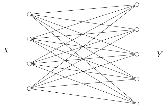
Obrázek 3.6: Graf G = \overset{\leftrightarrow}{K}_{\frac{n-1}{2}, \frac{n+1}{2}} , kde n = 9 . Každá neorientovaná hrana zde představuje dvě protichůdné orientované hrany mezi týmiž vrcholy.
