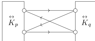
Obrázek 4.1: Silně 2-souvislý orientovaný graf s nezávislostí \alpha_2(G) = 2 , který není hamiltonovský.
