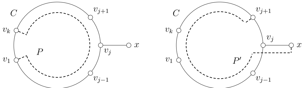
Obrázek 3.2: Situace z důkazu Diracovy věty. Čárkovaně je naznačena možná struktura cest P a P' .
