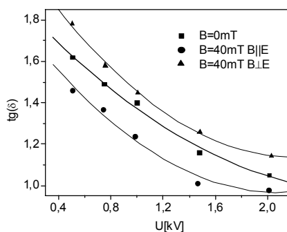
Obr. 5: Závislosť stratového činiteľa od priloženého napätia pri vysokej koncentracii (3,214%) magnetitových častíc.
