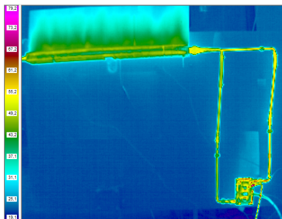
Obr. 3: Termovízny obraz odvodu tepla z IGBT prvku slučkovým termosyfónom.
